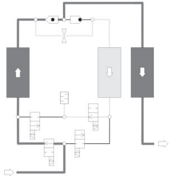
Adsorptie in de linker droogmiddeltank
