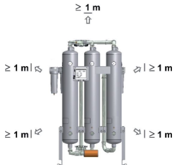
Vereiste afstand bovenaan en aan de zijkanten = min. 1 m
