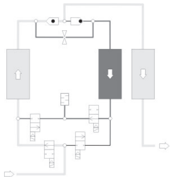
Regeneratie in de rechter droogmiddeltank
